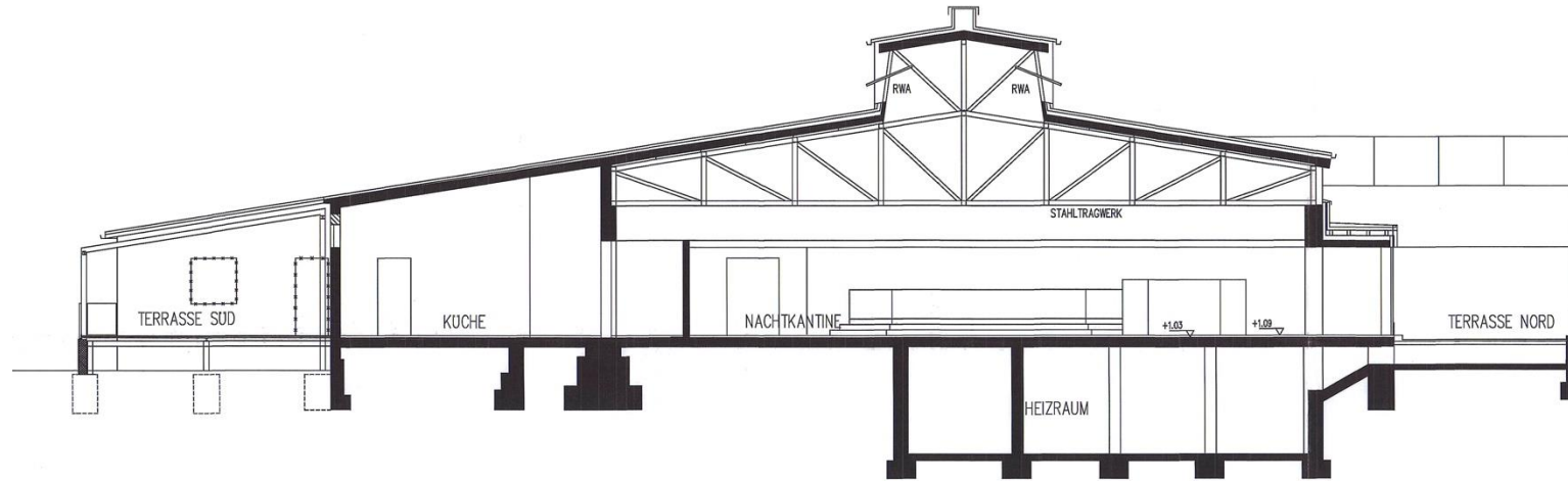
SCHNITT A-A
